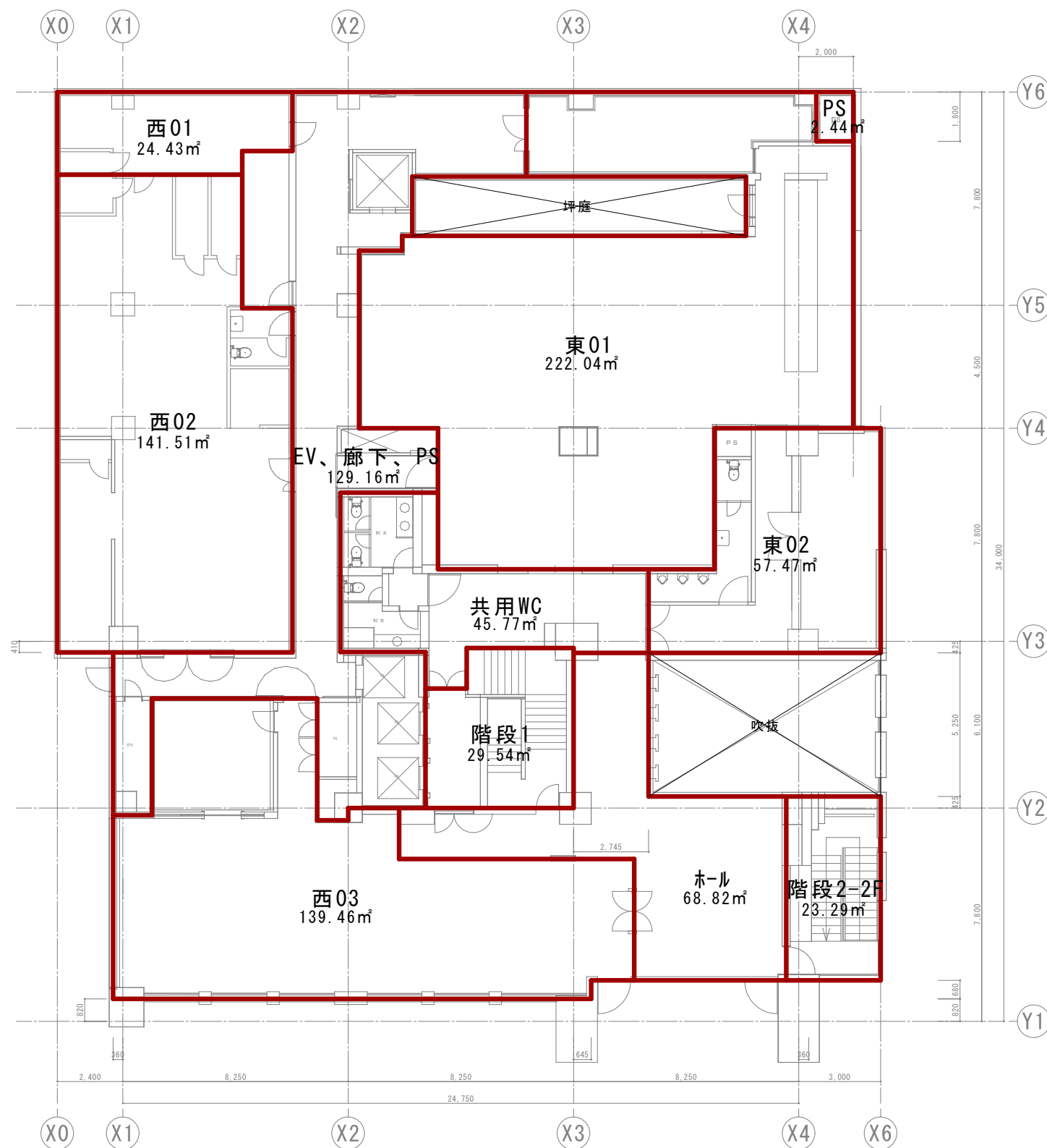
2階平面図
